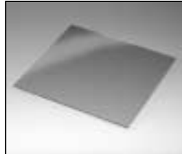
L4.82740.E Protection glass frosted from ser. no. 426 to 552 (405x395x2,75mm) for use with L4.82732.E Schutzscheibe gefrostet ab Ser.Nr. 426 bis 552 (405x395x2,75mm) zum Gebrauch mit L4.82732.E
